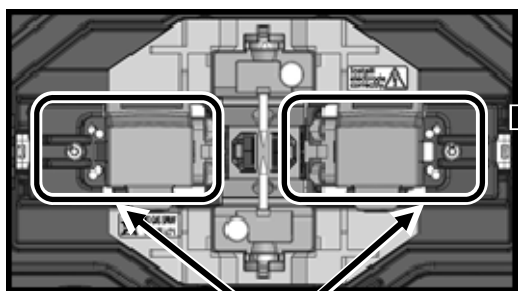
涂覆层光纤夹具
